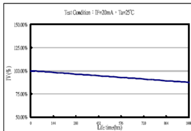
Fig6. Life Test at 20mA R.T. 1000hrs:
